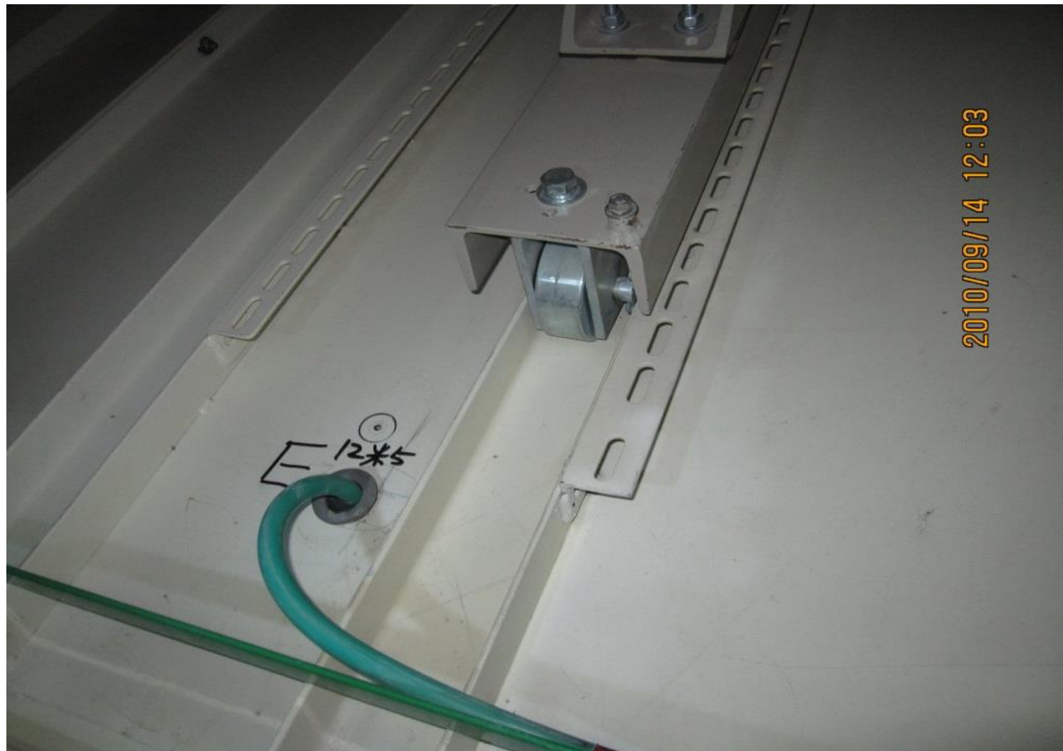
圖106工程會扣點編號5070427 說明：模鑄式變壓器輪子固定不當
