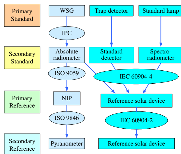
圖 2. 太陽光照射度偵測器基準設備和轉換方法校正追溯圖
