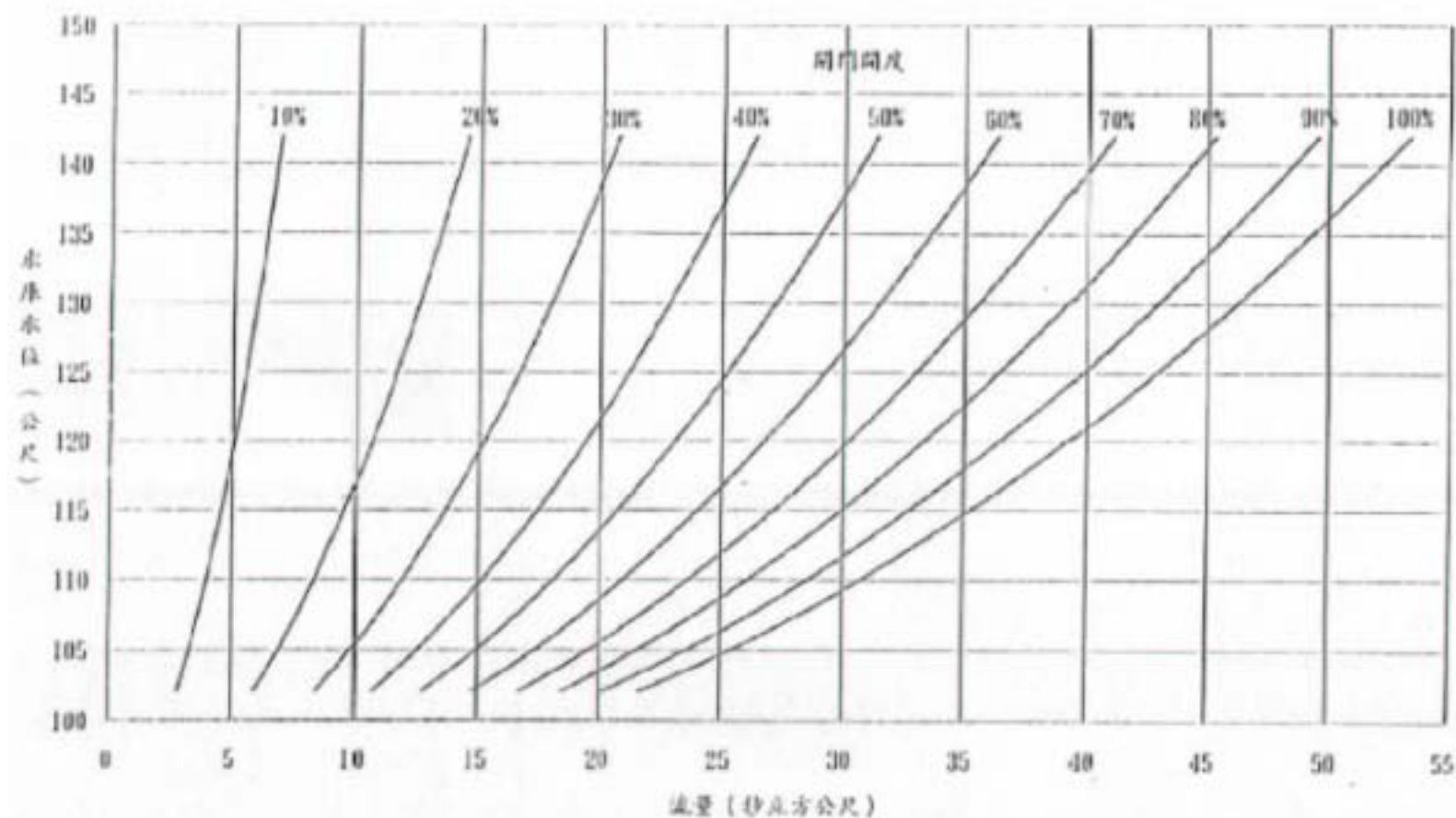
圖三：排水道控制閘門開度與放流量關係曲線
