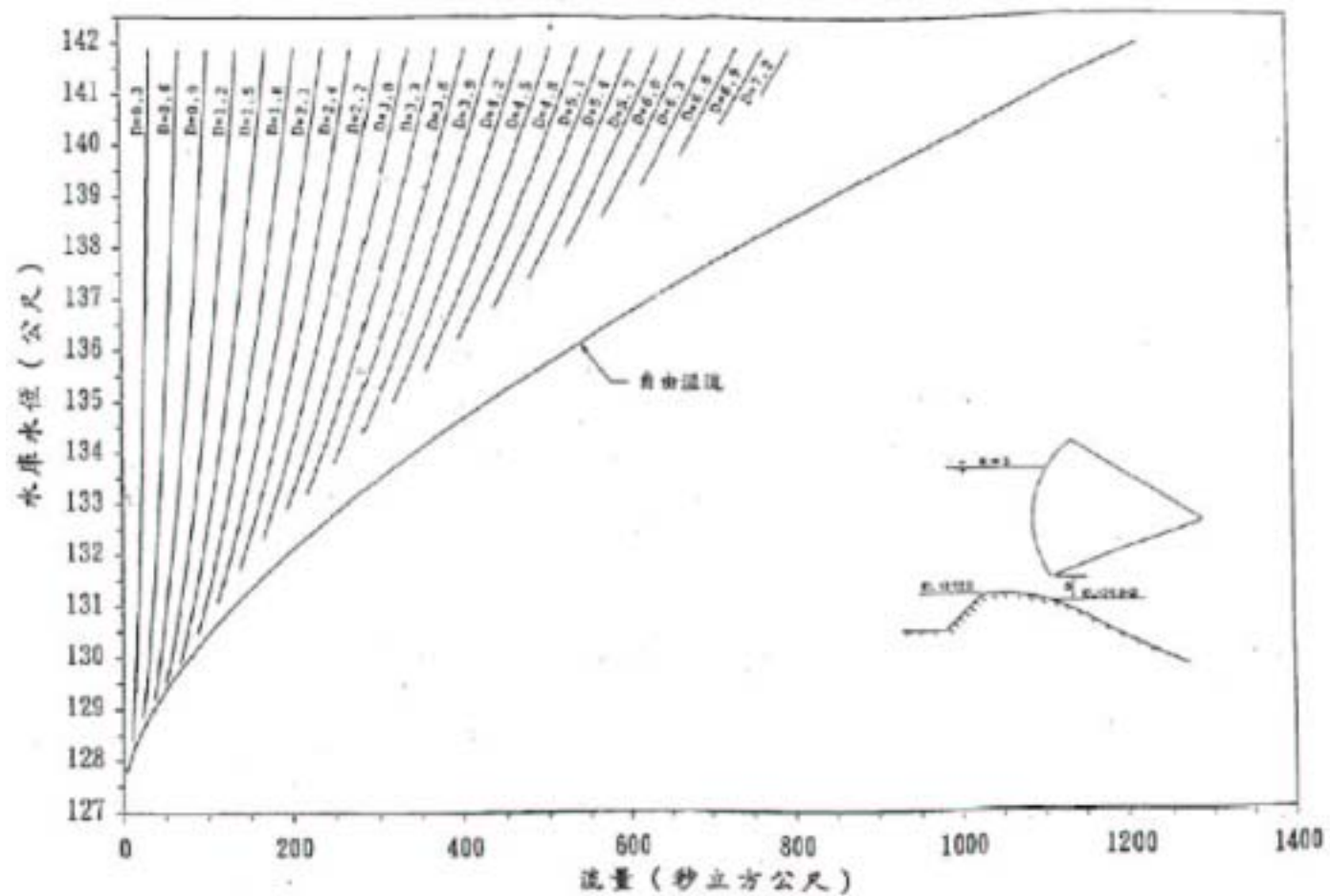
圖一：溢洪道閘門開度與放流量關係曲線（單門）
