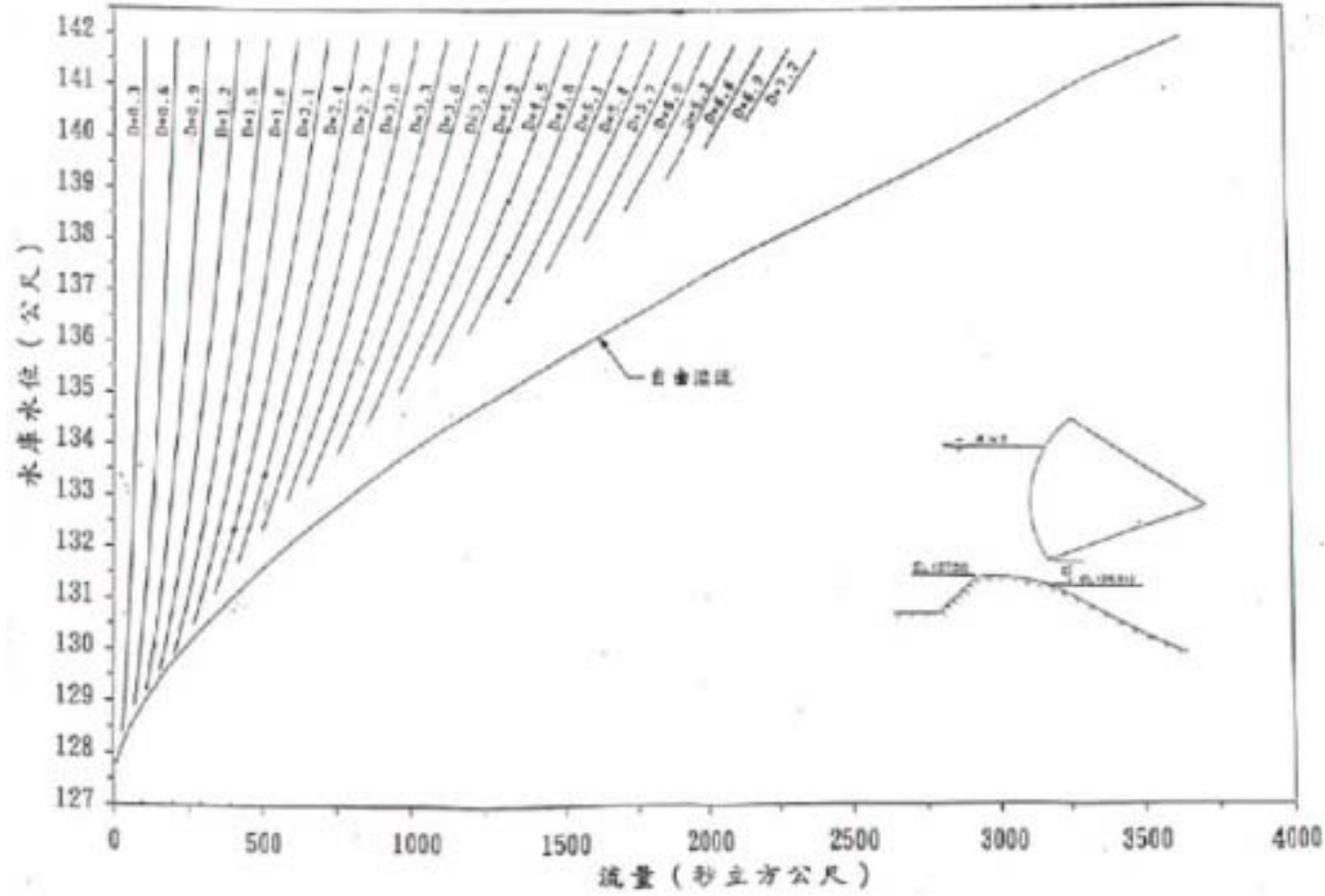
圖二：溢洪道閘門開度與放流量關係曲線（三門）
