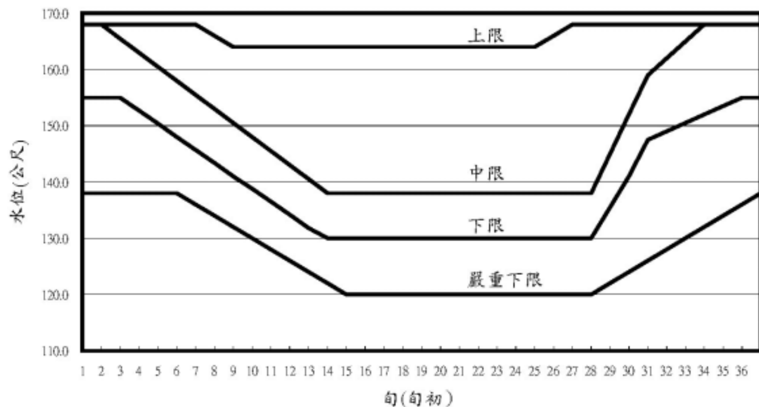
附圖一、翡翠水庫運用規線
