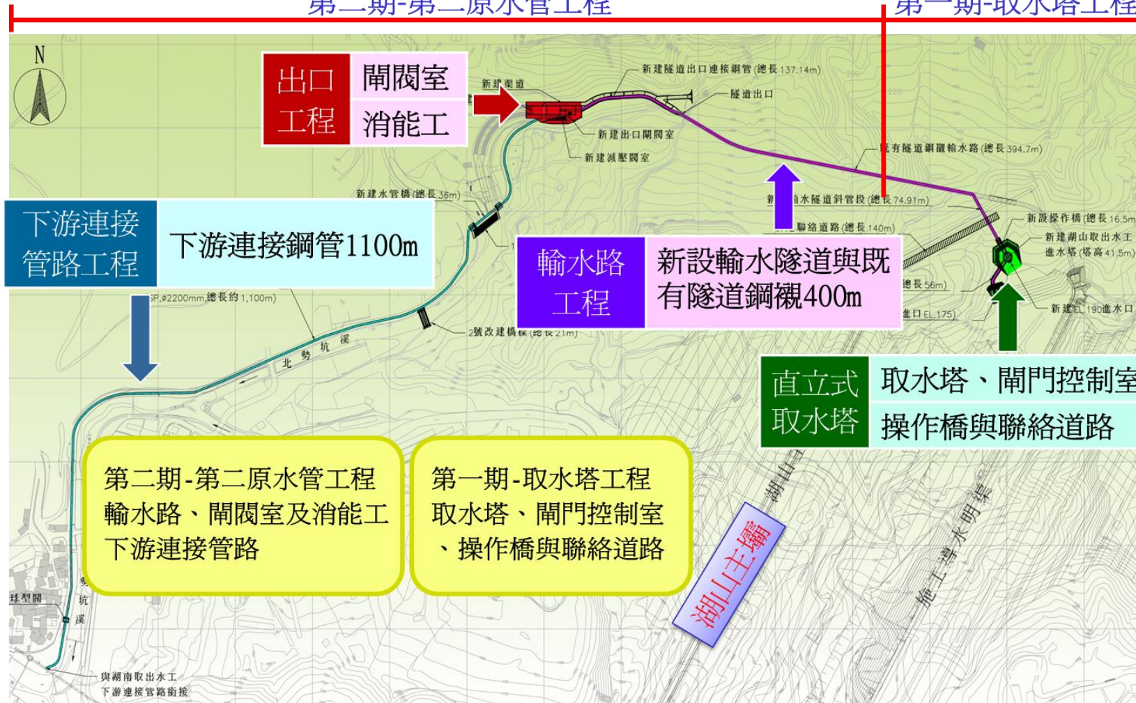
圖 4-1 湖山水庫第二原水管工程示意圖
